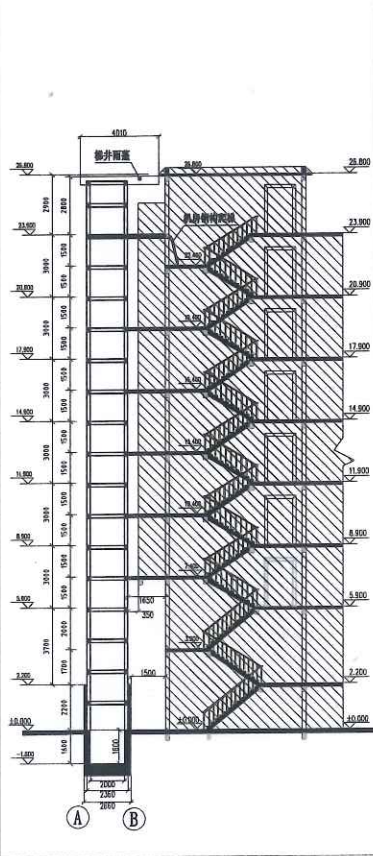
I-I剖面图
