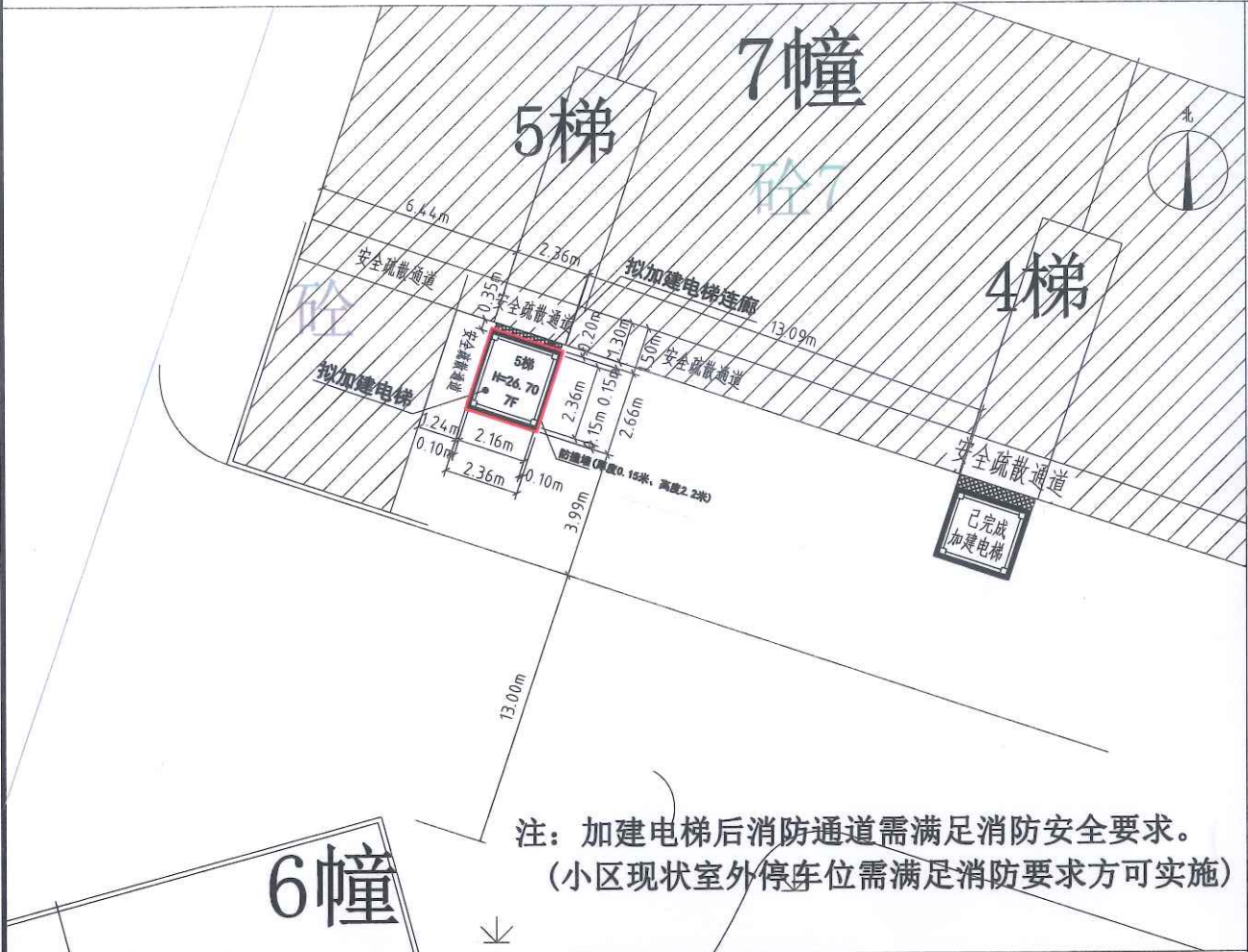
总平面图
