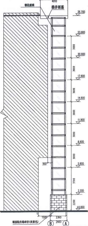
B-A轴立面图
