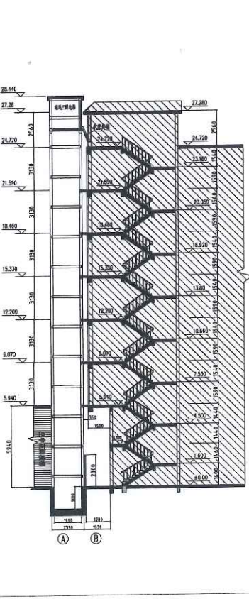
I-I剖面图
