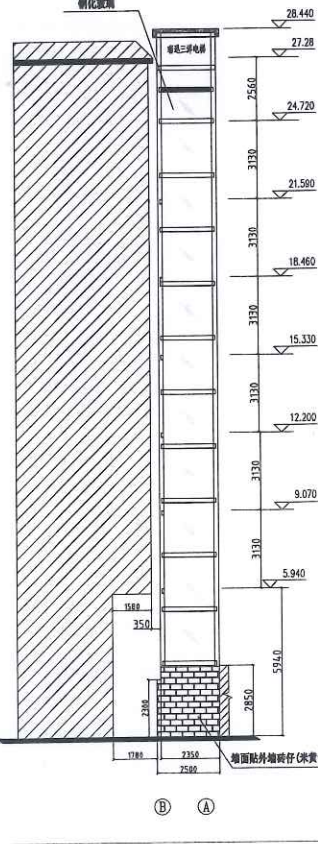
B-A轴立面图
