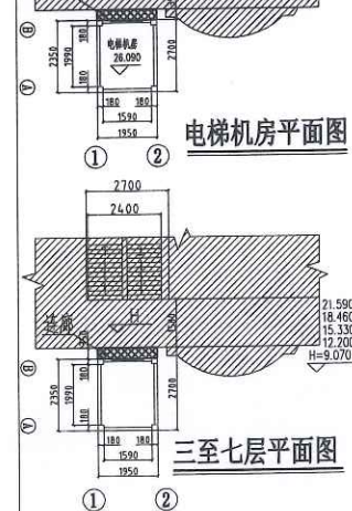
平面图2
